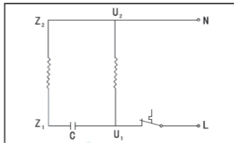
Grandinės schema
